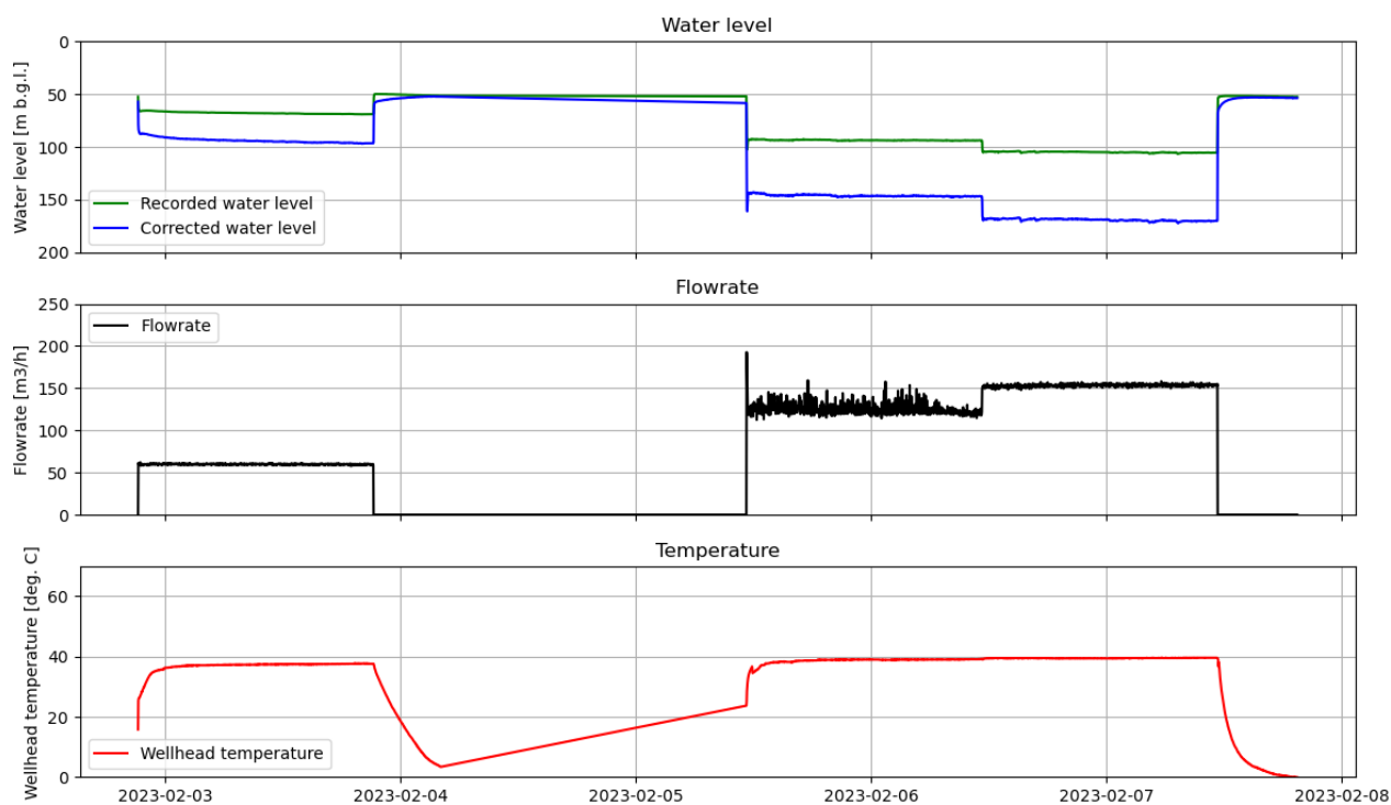
Fig. 2. Efekt zastosowania skryptu THERMALIFT CALC dla testu hydrodynamicznego wykonanego w jednym z otworów na Niżu Polskim
